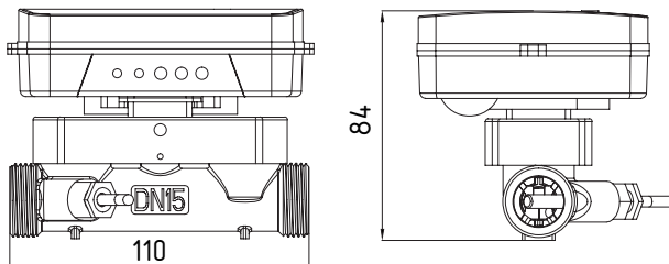
БЕРИЛЛ СТЭУ41.15-1,5-2...
