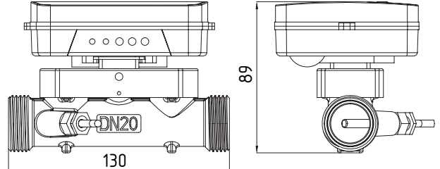
БЕРИЛЛ СТЭУ 41.20-2,5-2...
