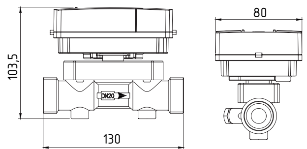
БЕРИЛЛ СТЭУ 41.20-2,5-1...
