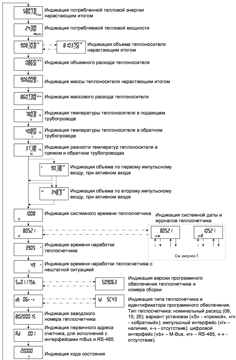
Рисунок 1. Последовательность переключения параметров на индикаторе теплосчетчика
